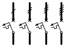
ΜΙΚΡΟΑΥΤΟΜΑΤΟΣ ΔΙΑΚΟΠΤΗΣ 1 Η΄ 2 Η΄ 3 Η΄ 4 ΠΟΛΩΝ
