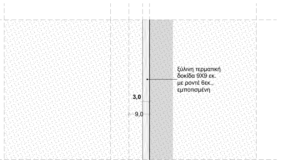
AP.E2: ARMOS EULINOS, TEΛΕΙΩΜΑ ΠΑΤΗΜΕΝΟ ΧΩΜΑ - ΕΛΕΥΘΕΡΟ ΤΕΛΕΙΩΜΑ ΚΑΤΩΨΗ
