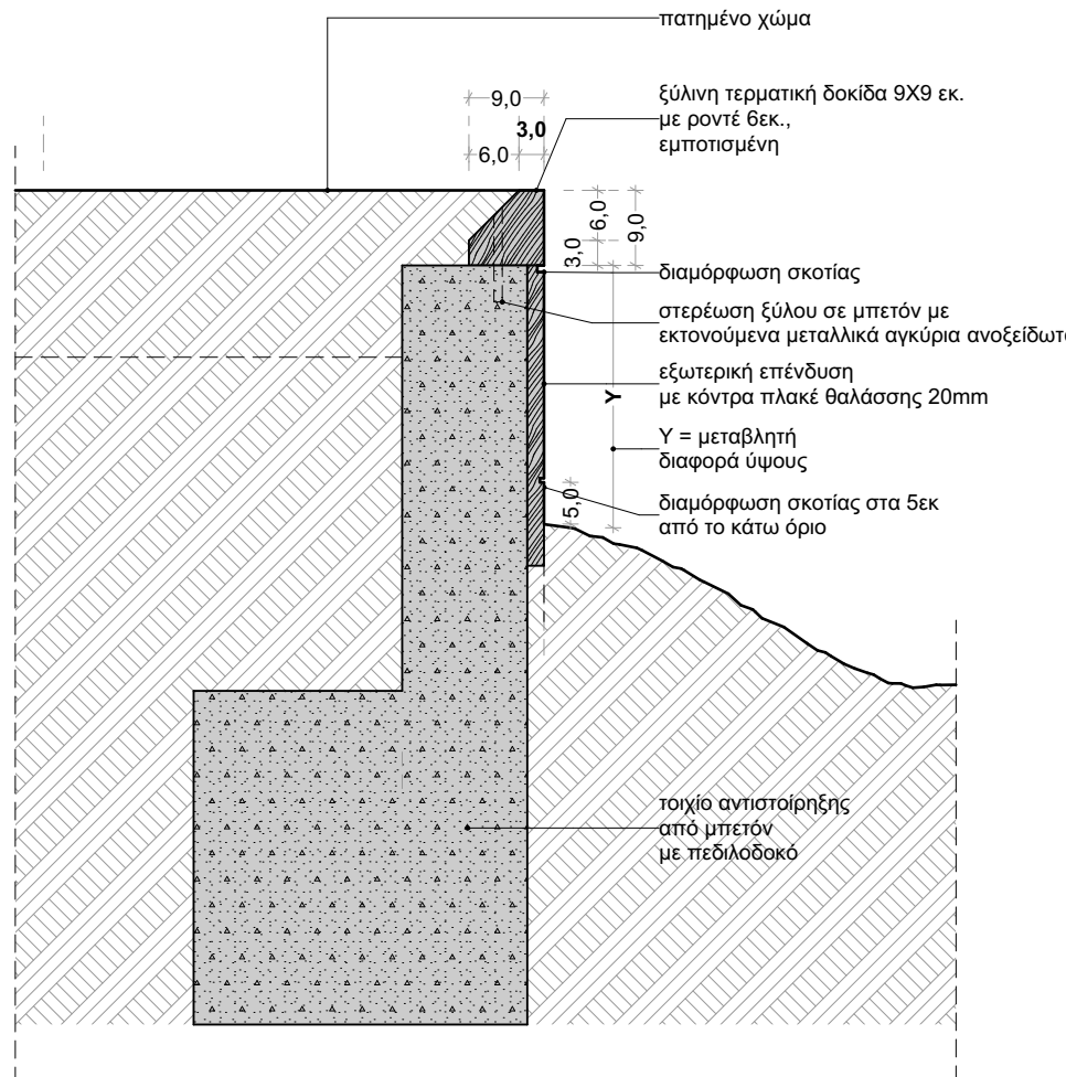
AP.E2: ARMOS EULINOS, TEΛΕΙΩΜΑ ΠΑΤΗΜΕΝΟ ΧΩΜΑ - ΕΛΕΥΘΕΡΟ ΤΕΛΕΙΩΜΑ ΤΟΜΗ
