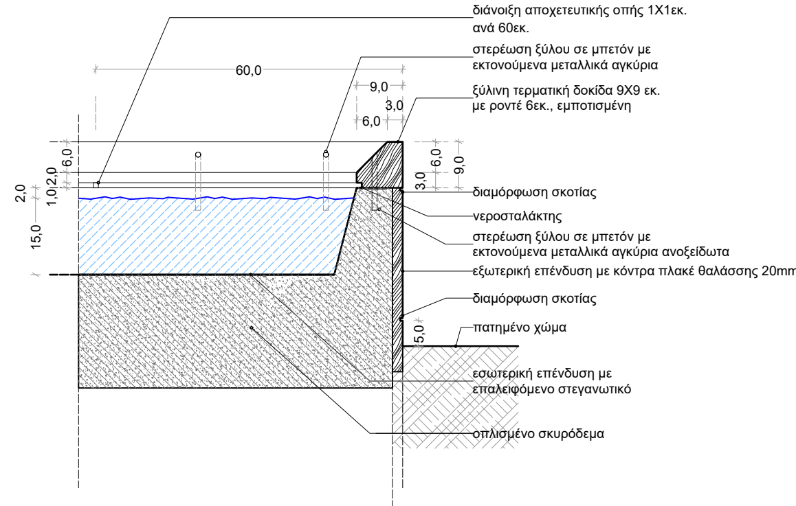
AP.E4: ΣΤΟΙΧΕΙΟ ΝΕΡΟΥ ΣΥΝΑΡΜΟΓΗ ΜΕ ΠΑΤΗΜΕΝΟ ΧΩΜΑ ΤΟΜΗ
