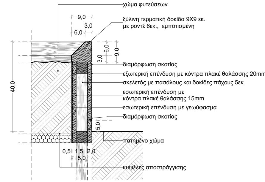
AP.E3: ΖΑΡΠΤΙΝΙΕΡΑ ΣΥΝΑΡΜΟΓΗ ΜΕ ΠΑΤΗΜΕΝΟ ΧΩΜΑ ΤΟΜΗ
