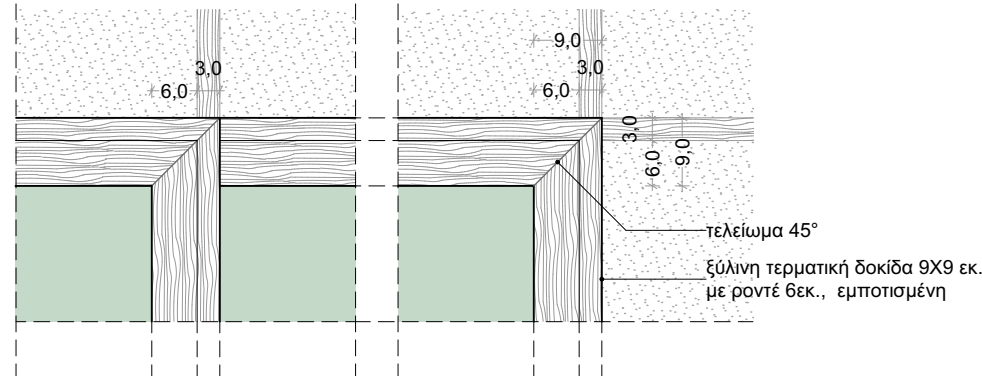
AP.E3: ΖΑΡΠΤΙΝΙΕΡΑ ΣΥΝΑΡΜΟΓΗ ΜΕ ΖΑΡΠΤΙΝΙΕΡΑ ΚΑΤΩΨΗ
