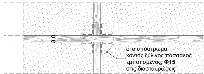
AP.E1: ARMOS EULINOS ΣΥΝΑΡΜΟΓΗ ΜΕ ΠΑΤΗΜΕΝΟ ΧΩΜΑ ΚΑΤΩΨΗ
