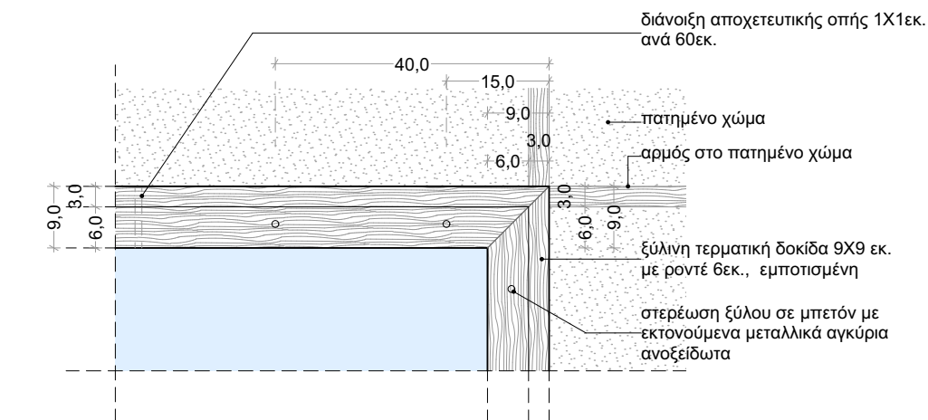
AP.E4: ΣΤΟΙΧΕΙΟ ΝΕΡΟΥ ΣΥΝΑΡΜΟΓΗ ΜΕ ΠΑΤΗΜΕΝΟ ΧΩΜΑ ΚΑΤΩΨΗ
