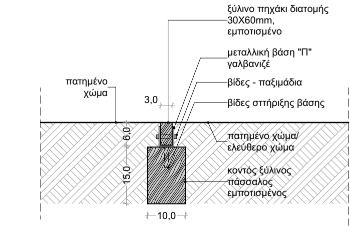
AP.E1: ARMOS EULINOS ΣΥΝΑΡΜΟΓΗ ΜΕ ΠΑΤΗΜΕΝΟ ΧΩΜΑ ΤΟΜΗ
