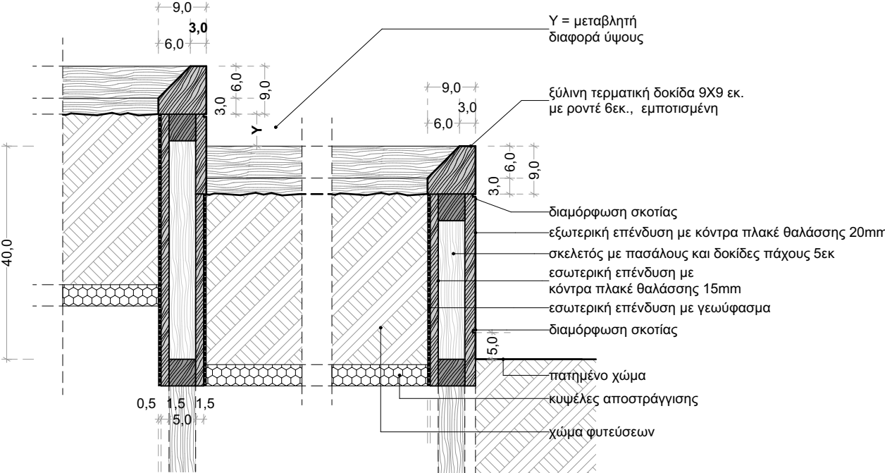
AP.E3: ΖΑΡΠΤΙΝΙΕΡΑ ΣΥΝΑΡΜΟΓΗ ΜΕ ΖΑΡΠΤΙΝΙΕΡΑ ΤΟΜΗ
