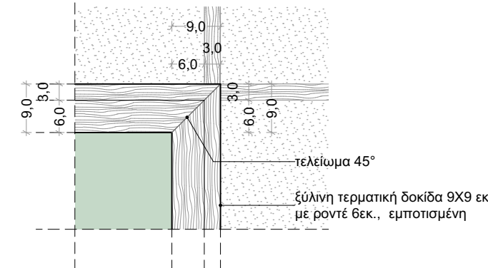
AP.E3: ΖΑΡΠΤΙΝΙΕΡΑ ΣΥΝΑΡΜΟΓΗ ΜΕ ΠΑΤΗΜΕΝΟ ΧΩΜΑ ΚΑΤΩΨΗ
