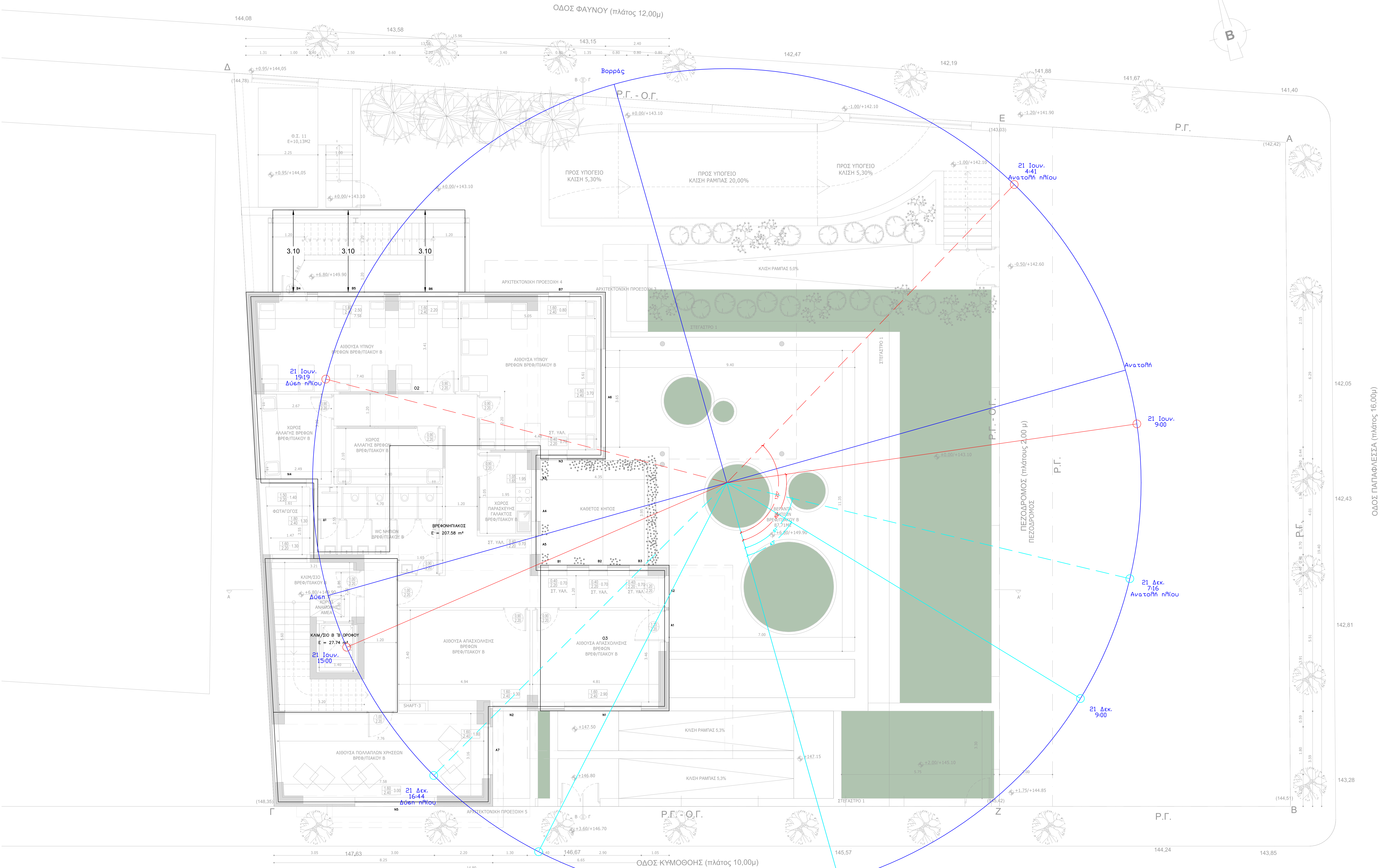
ΚΑΤΩΗ Β' ΟΡΟΦΟΥ ΚΛΙΜΑΚΑ 1:50
